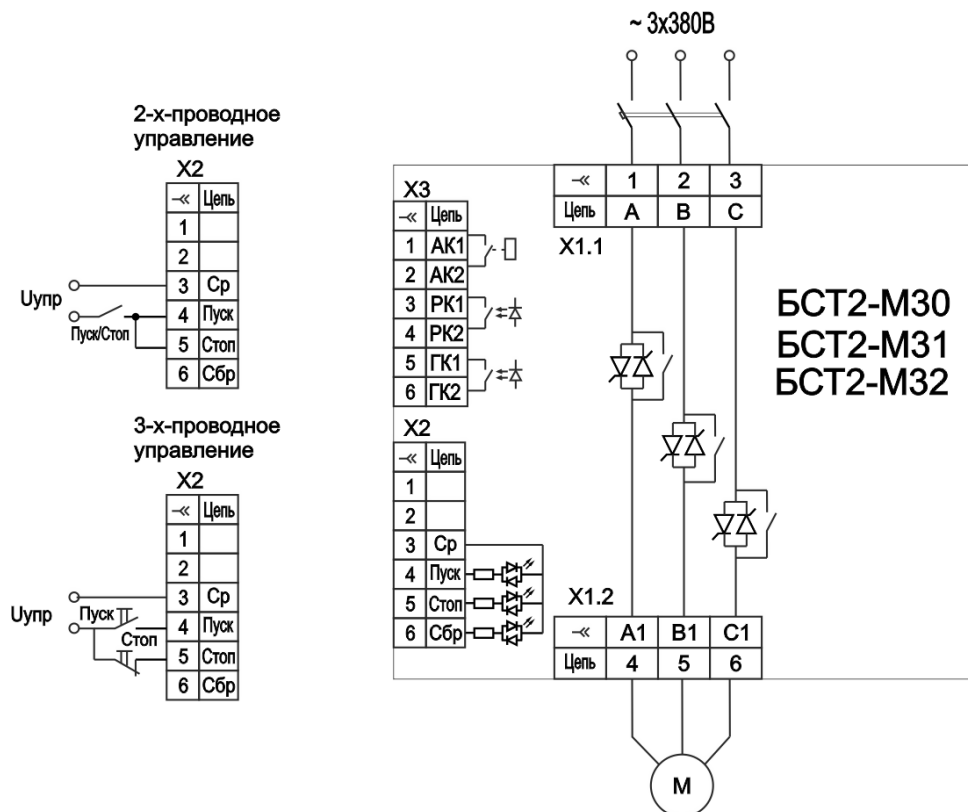
Рисунок 3 – Пример схемы подключения БСТ2-М30, БСТ2-М31, БСТ2-М32
