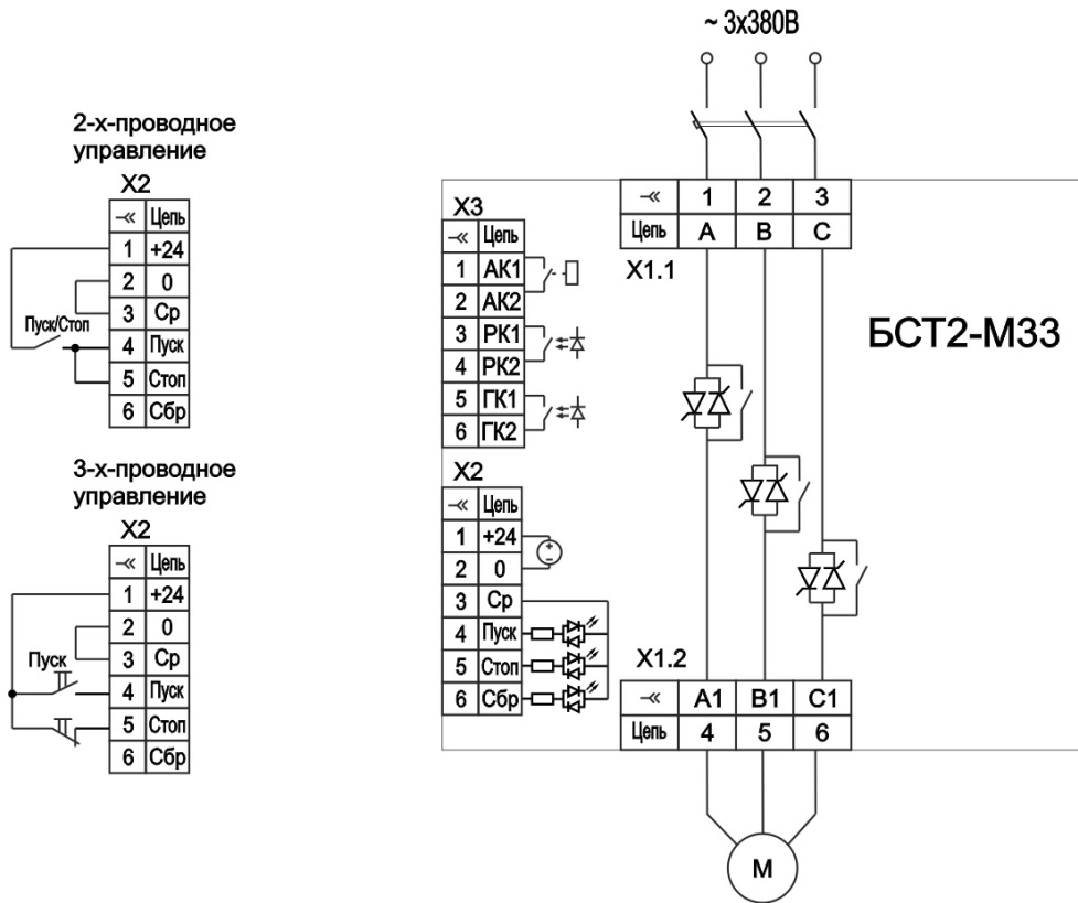
Рисунок 4 – Пример схемы подключения БСТ2-М33
