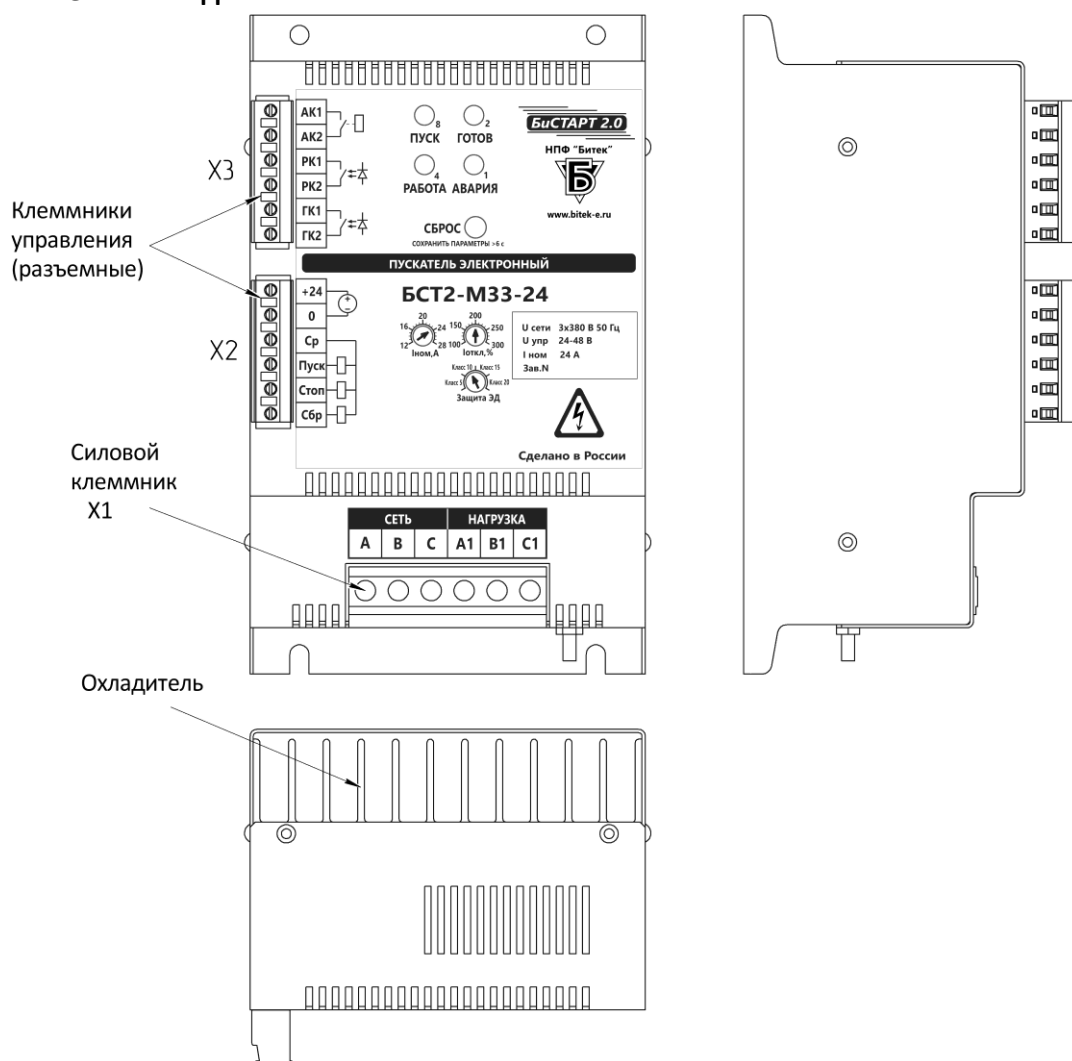
Рисунок 1 - Внешний вид пускателя БСТ2-М33-24
